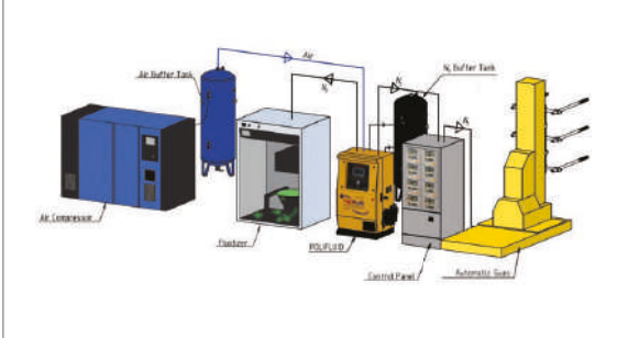
LINEA COMBINATA CON 2 RECIPROCATORI / COMBINED 2 ROBOTS LINE
